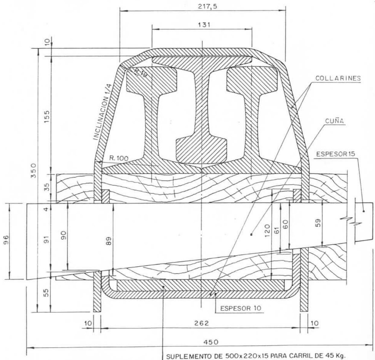
SECCION TRANSVERSAL
