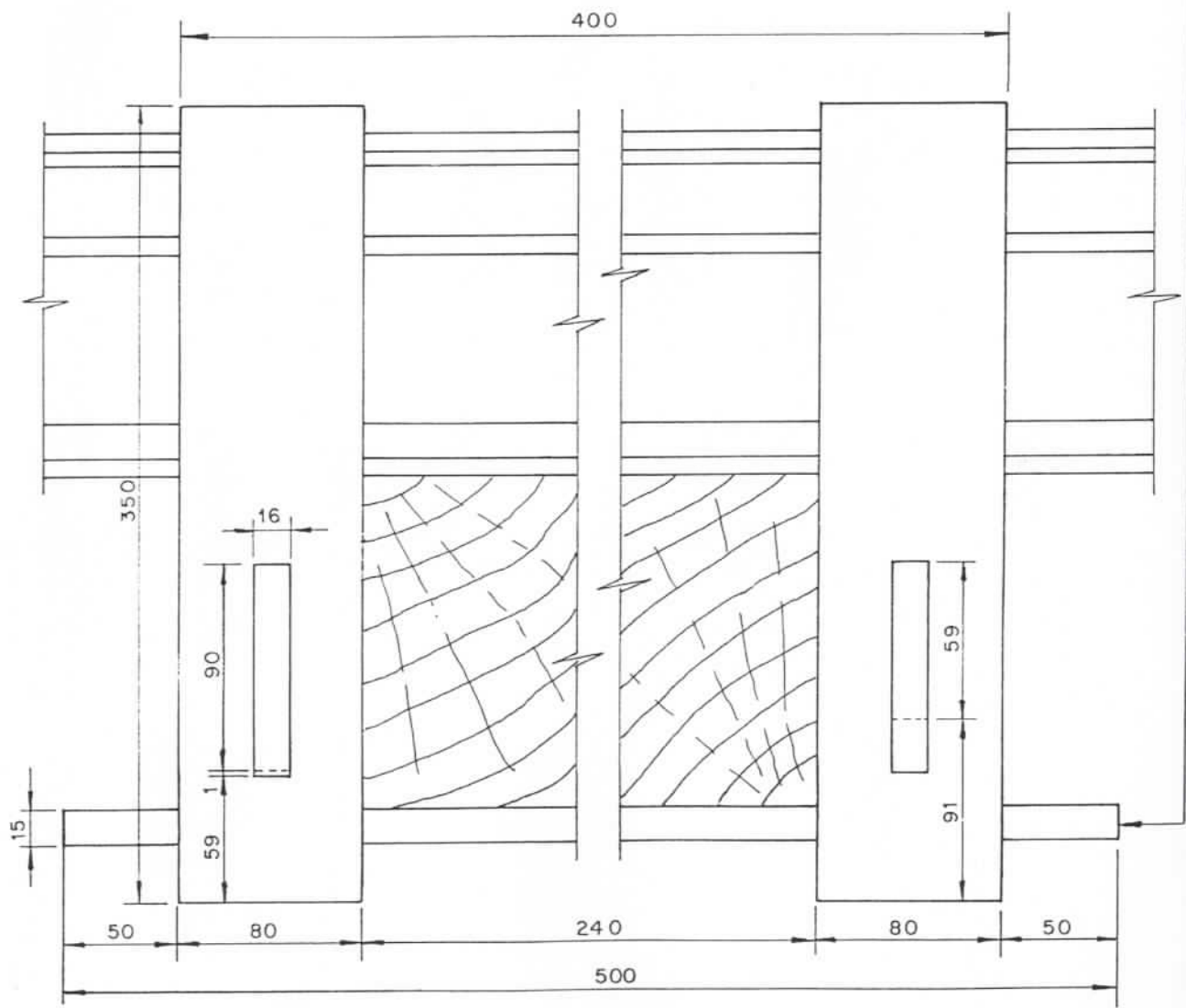
ALZADO LONGITUDINAL
