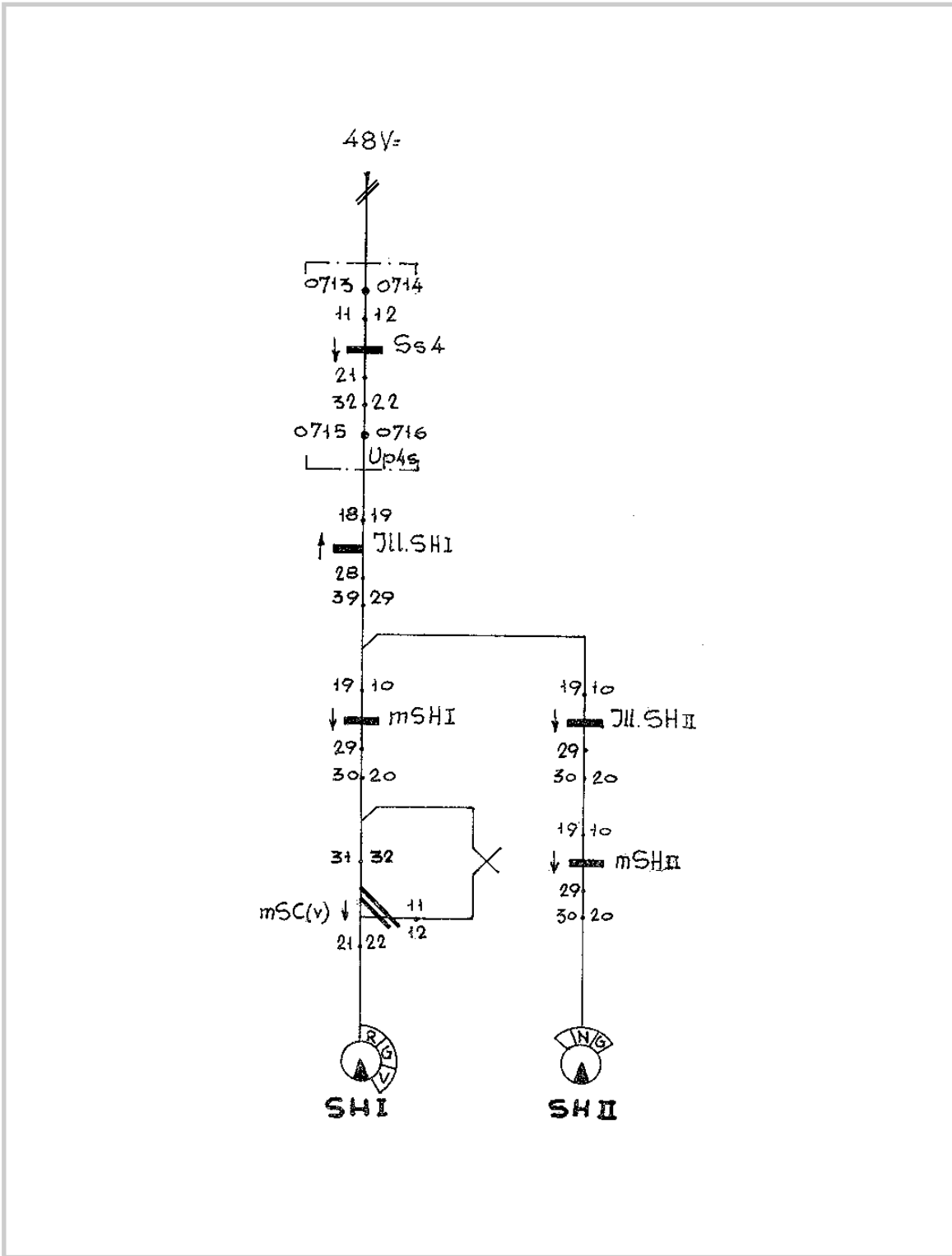
Tav. 2 Esempio di uno schema di circuito per manovra segnali
