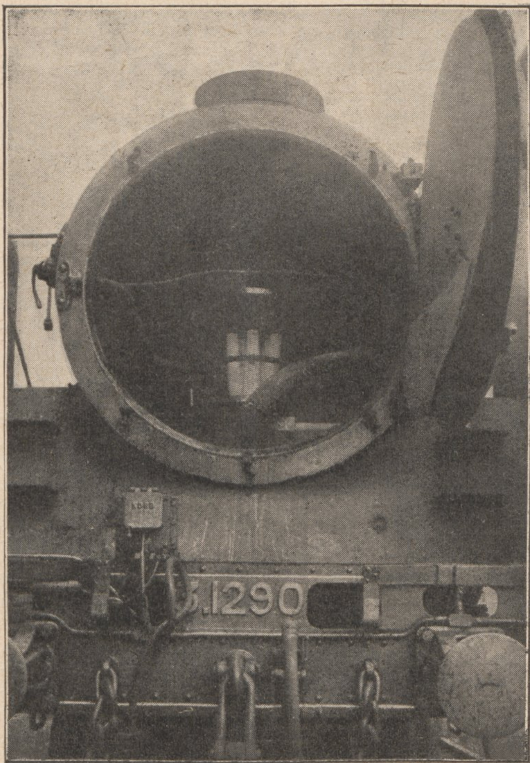
Fig. 8. — Echappement Lemaitre-Nord appliqué aux locomotives Compound de la série 3.1251-90
