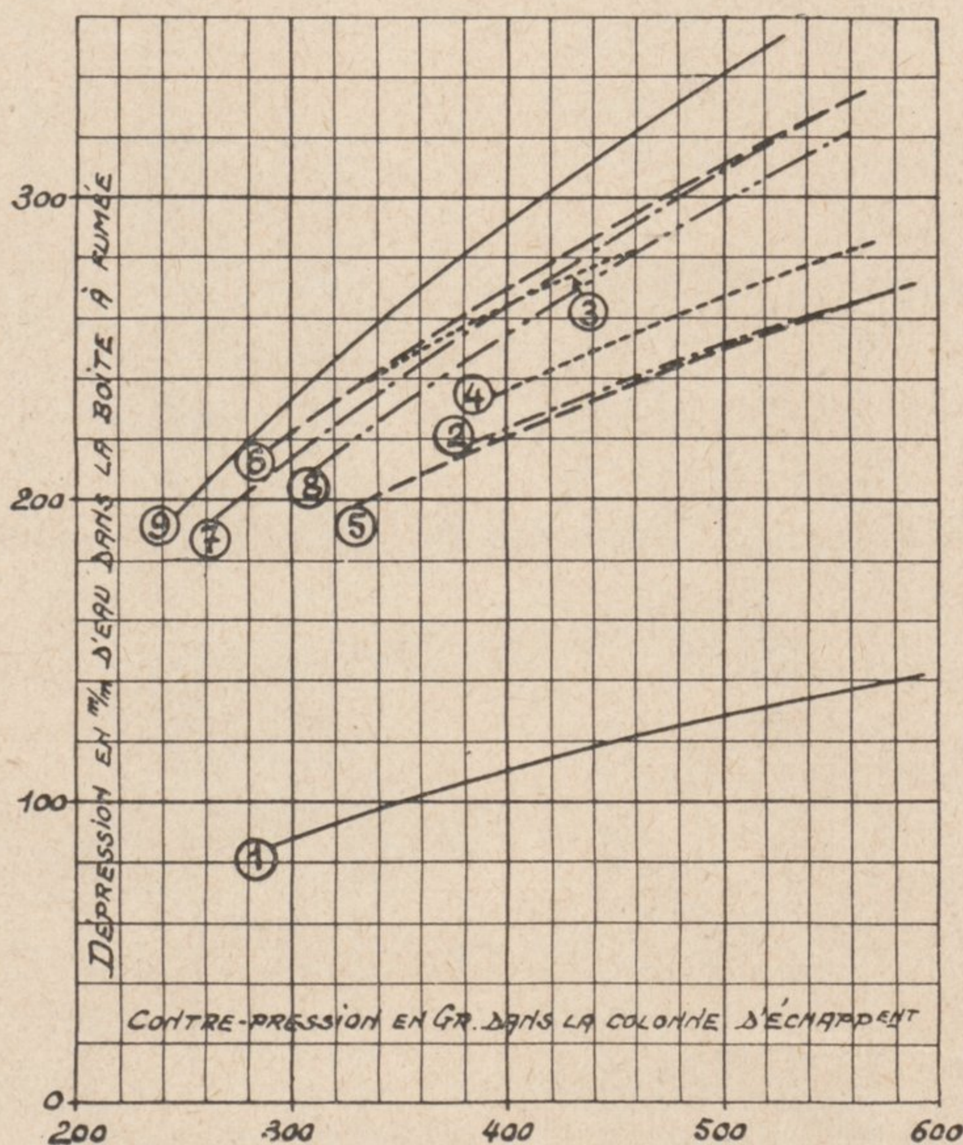
LOCOMOTIVE 3.1290 — COMPARAISON DES DÉPRESSIONS ET CONTRE-PRESSIONS DES DIVERS ÉCHAPPEMENTS AU CRAN 6
