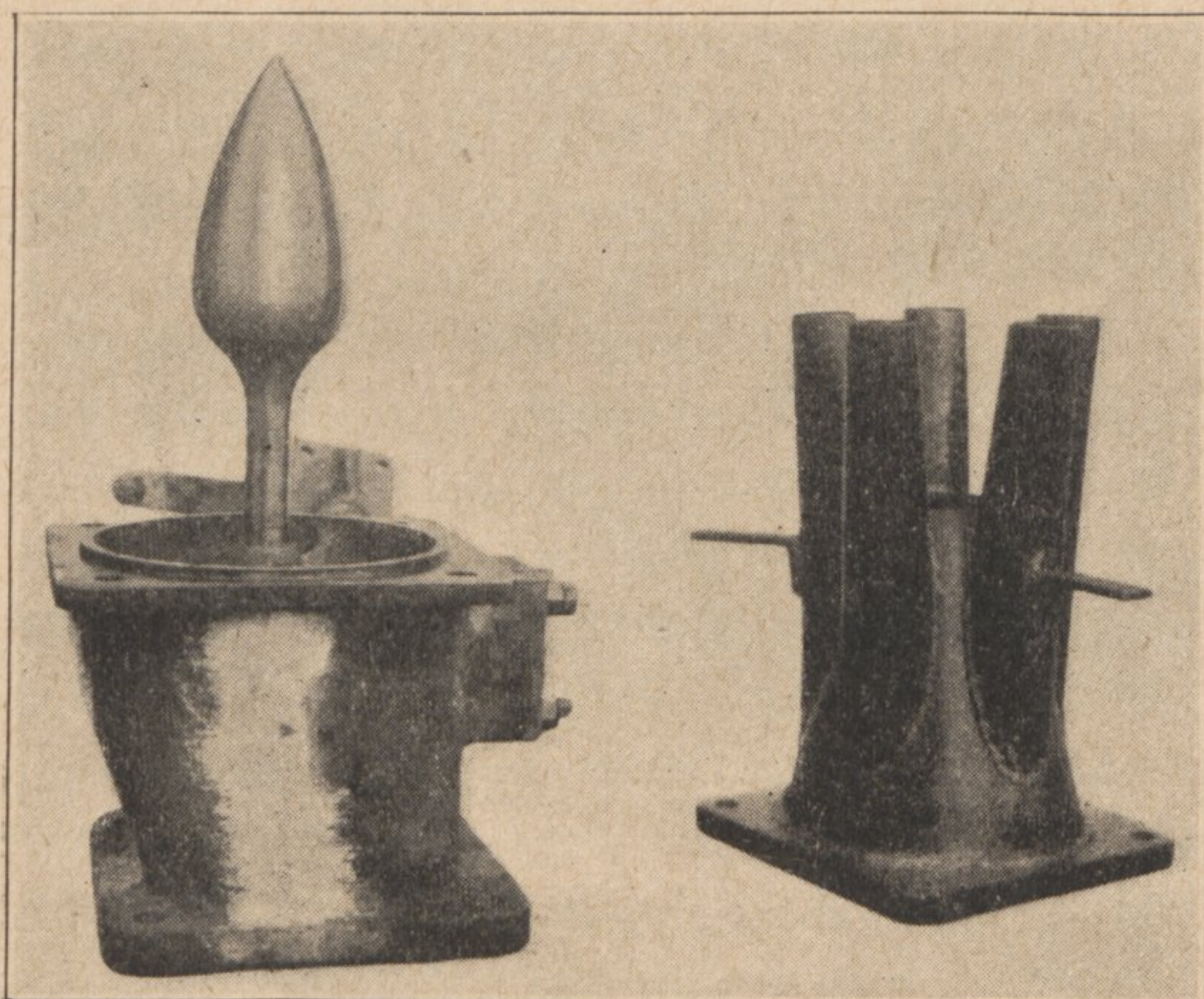
Fig. 2. — Dispositif variable de l'échappement Lemaître-Nord
