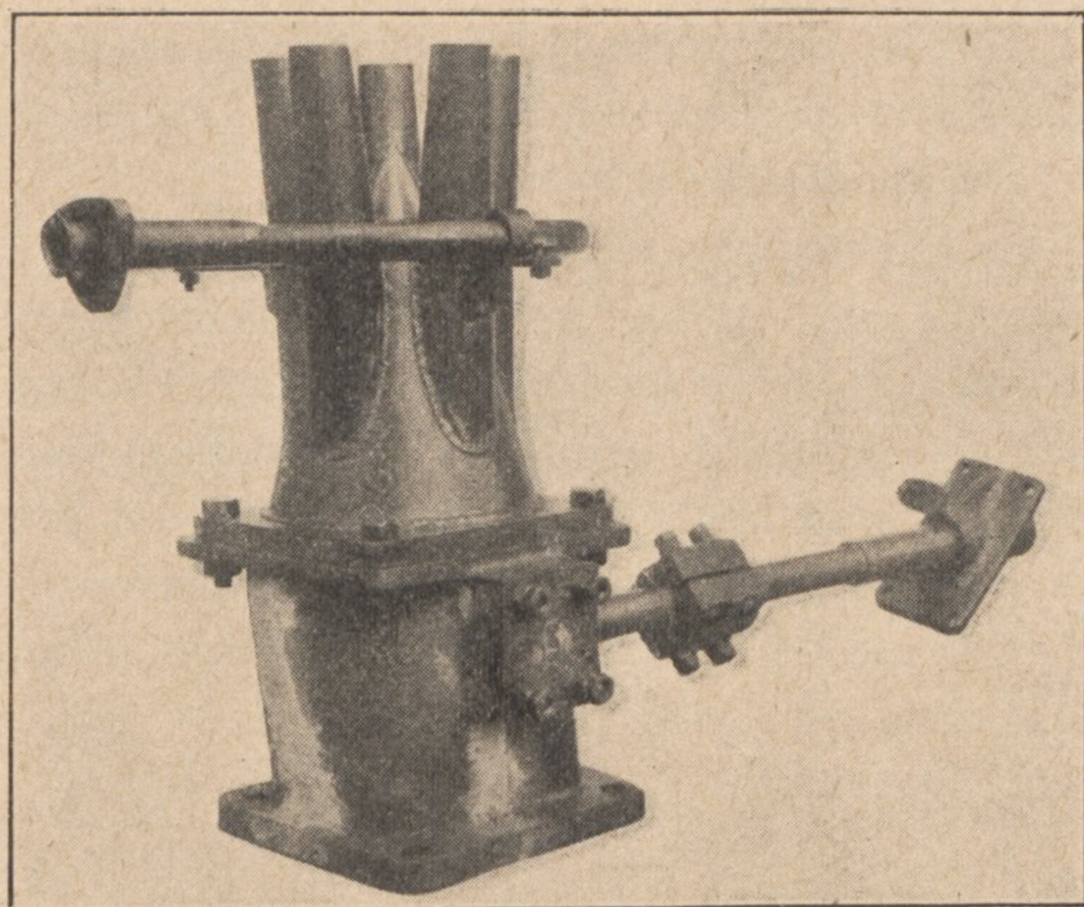
Fig. 1. — Tête d'échappement Lemaître-Nord à 5 tuyères
