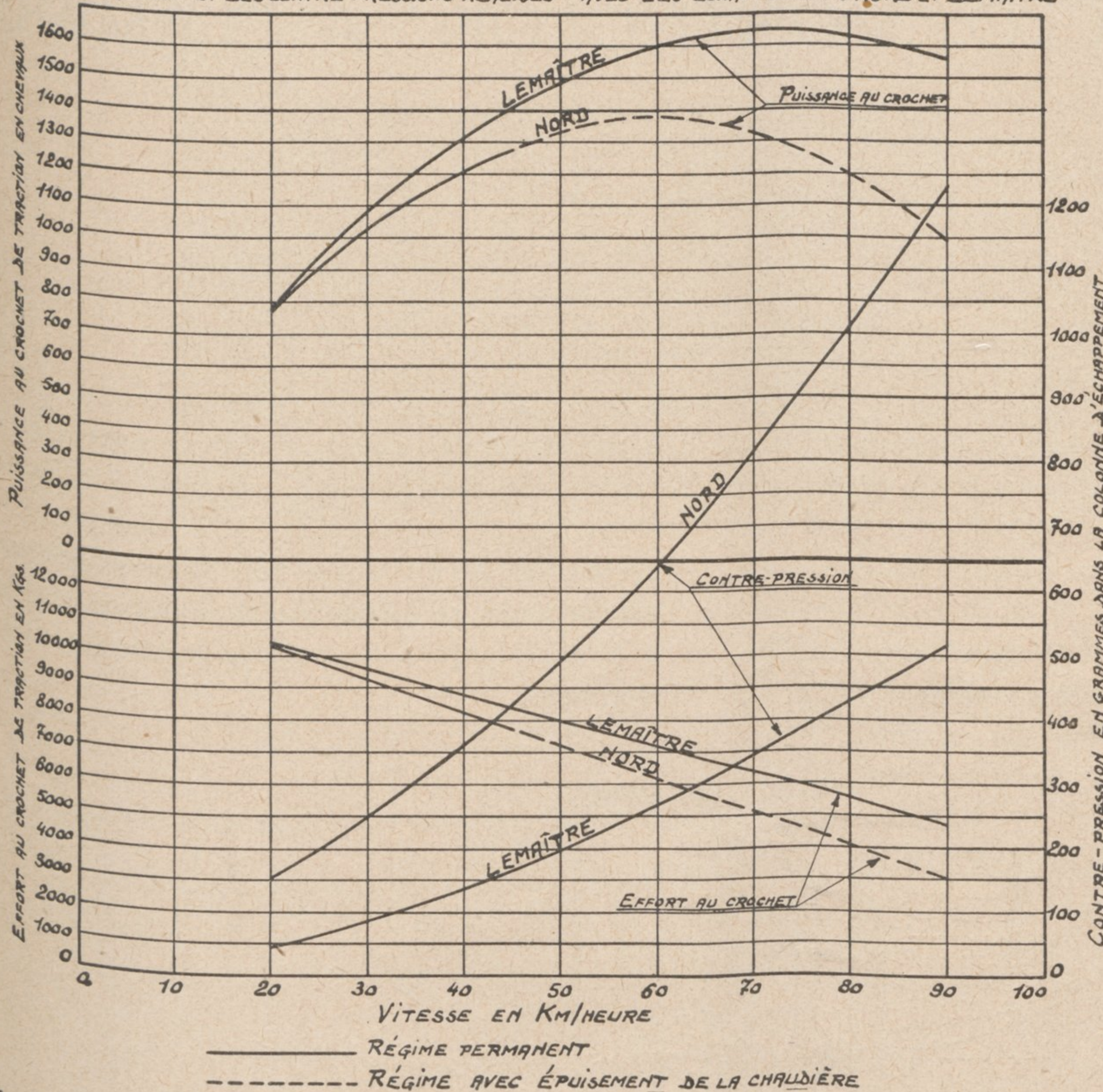
Figure 9 LOCOMOTIVE 4.192 - COMPARAISON DES PUISSANCES, DES EFFORTS AU CROCHET DE TRACTION ET DES CONTRE-PRESSIONS RÉALISÉS AVEC LES ÉCHAPPEMENTS "NORD" ET "LEMAÎTRE"
